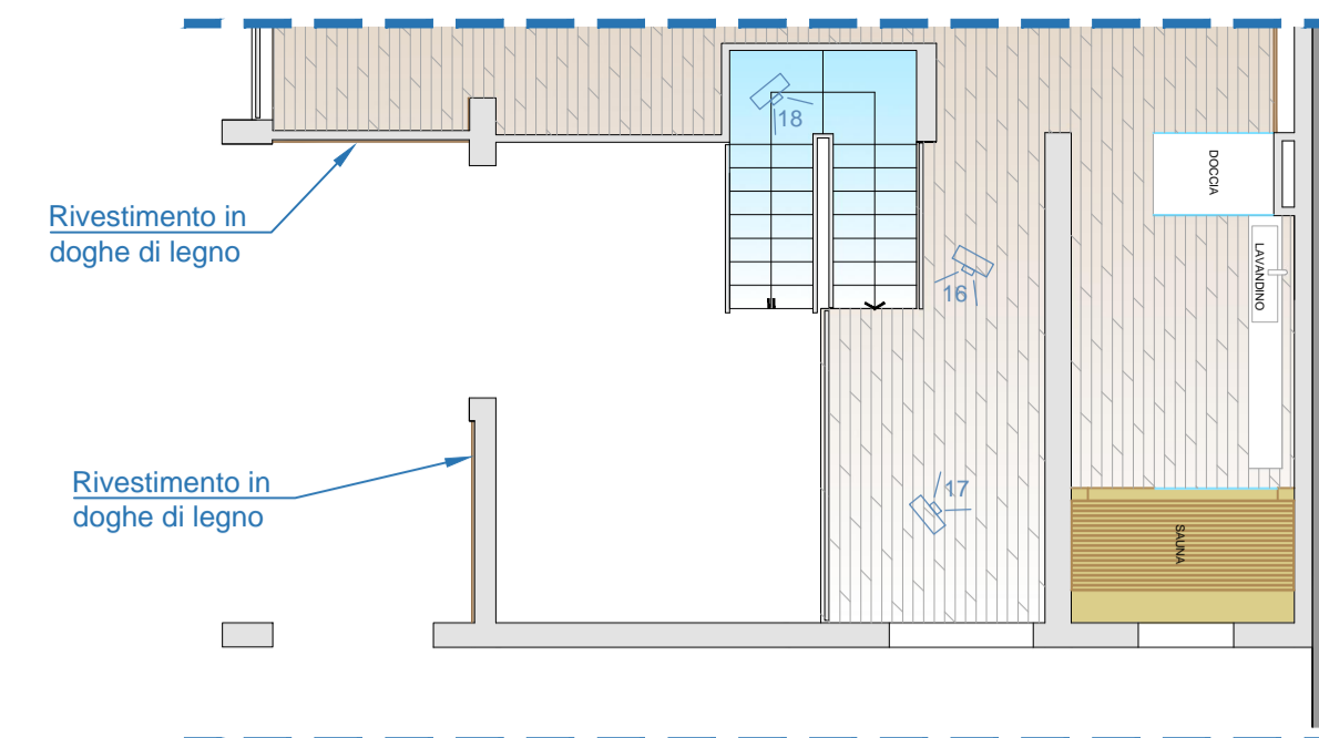
Pianta di riferimento 4 - primo
