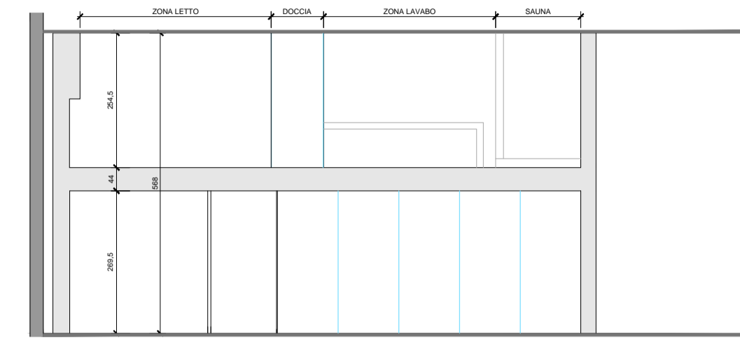
Sezione C-C
