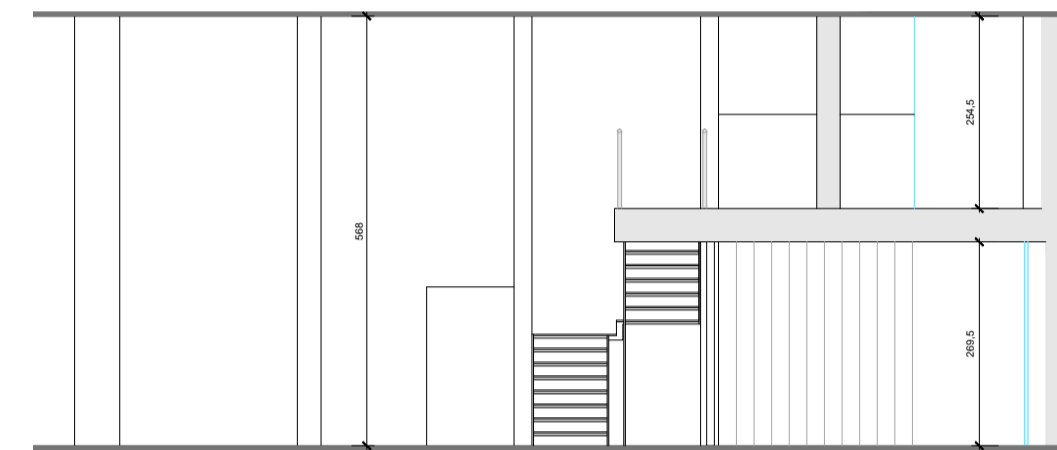
Sezione D-D
